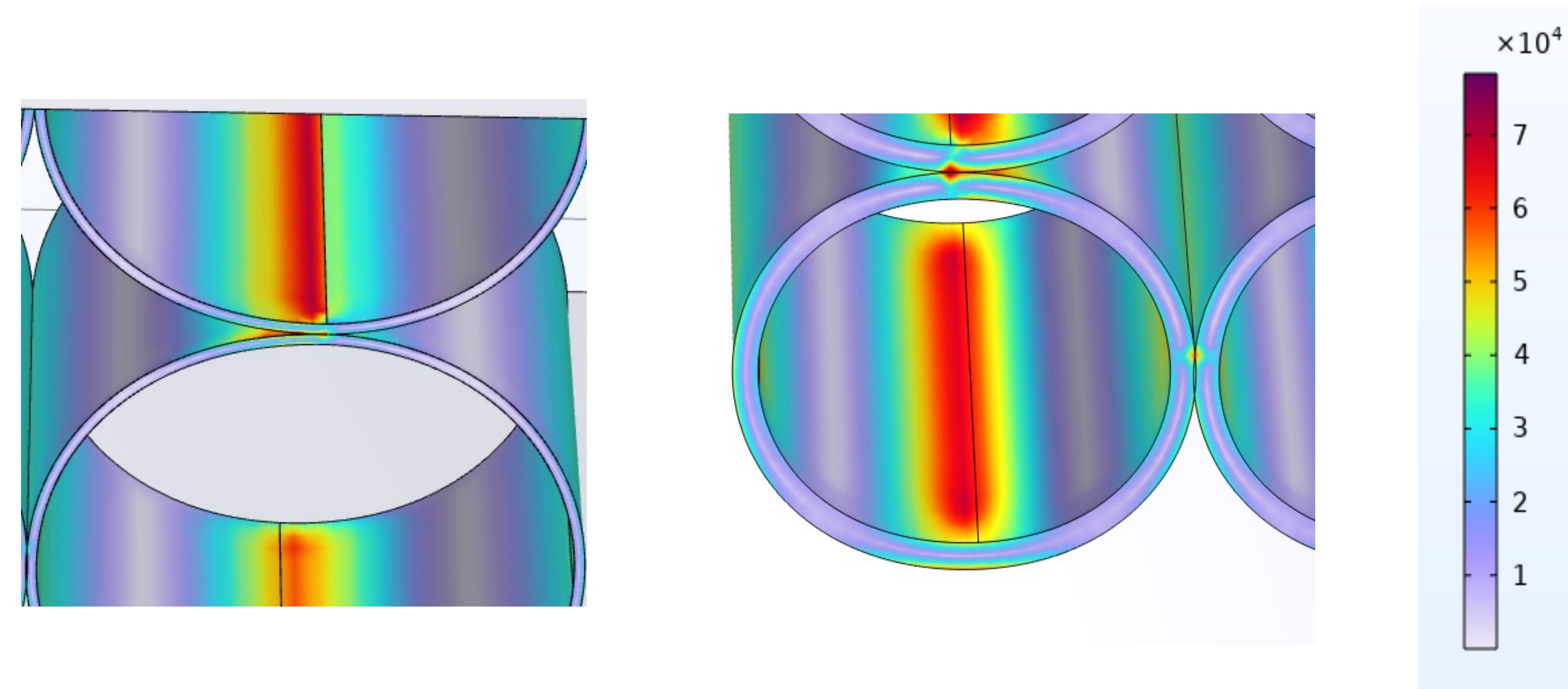
图 2. 左：壁厚度为0.01mm时应力情况； 右：壁厚度为0.03mm时应力情况。
